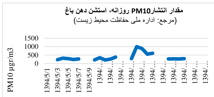
شکل (3) مقدار PM_{10} به میکروگرام درفی مترمکعب نظربه زمان های مختلف [3] جدول (2) گاز های گلخانه ای در شهر کابل به تن در سال توسط ADB، [4]
