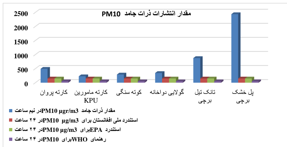
شکل (4) مقدار انتشارات ذرات جامد توسط پوهنتون پولی تخنیک کابل [3]
