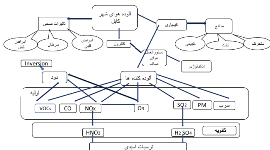
شکل ( ۱ ) وضعیت الوده گی هوای شهر کابل
