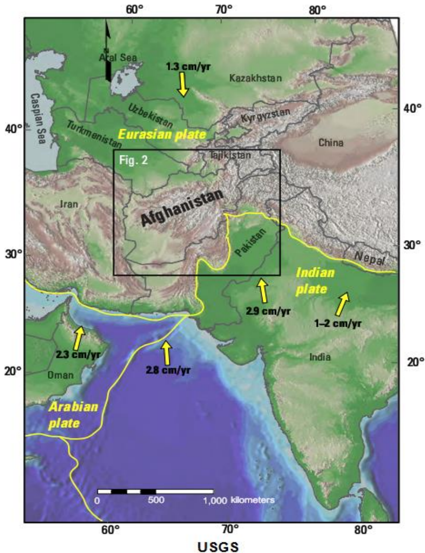
شکل ۲. سرعت حرکت صفحات هند، عرب و اروپایی-آسیا
