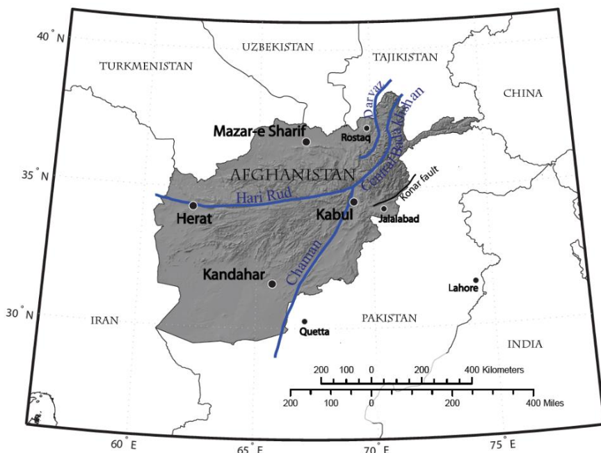
شکل ۵. موقعیت چهار شکست عمده در افغانستان (خط های بزرگ آبی)
