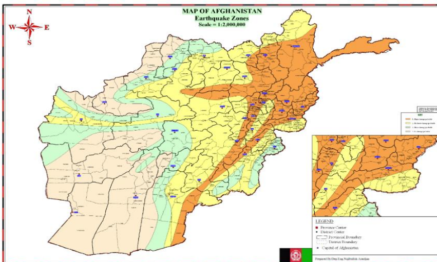
شکل ۳. نقشه زمین لرزه خیزی در
